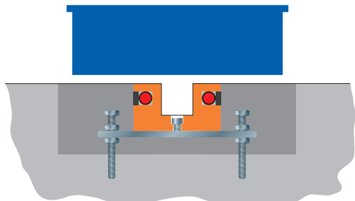
Kabel mit Führungsprofil verlegt
