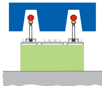
Kabel aufgeständert
