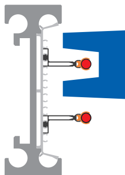
Kabel in einem EHB-Profil
