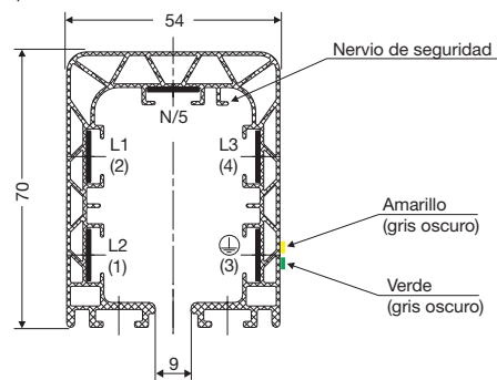
A - A KBH-5 polos
