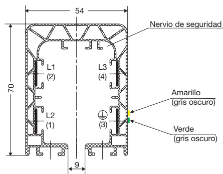
A - A KBH-4 polos
