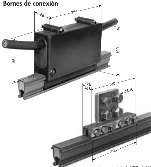
Montaje sobre un tramo de Carril
